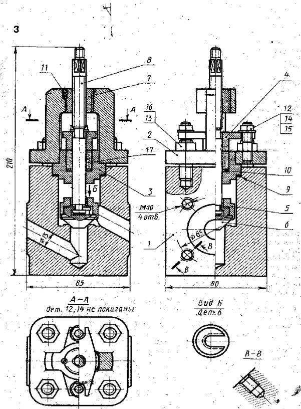
Рис. 43. Ветиль запорный
